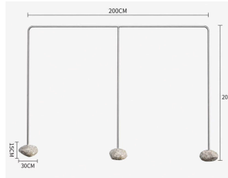
壁面がない店舗へ、中央脚を追加した自立ラックの提案図
